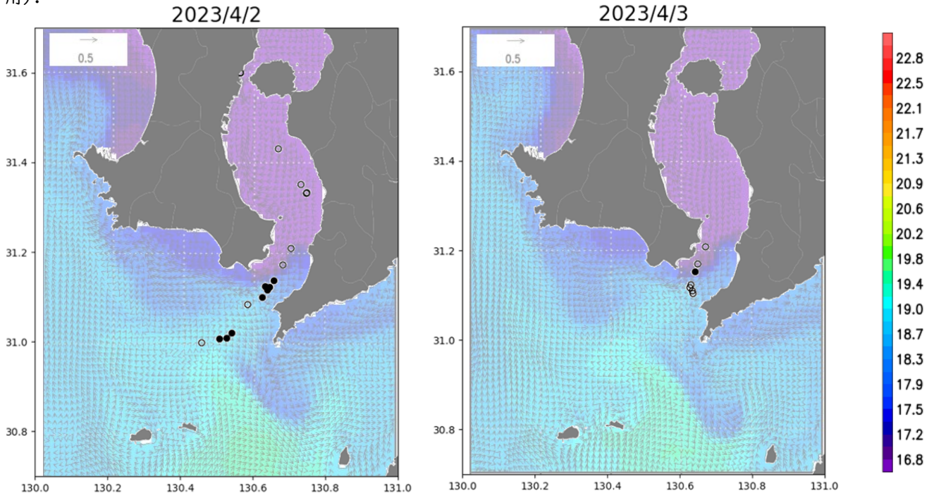
図2. 鹿児島大学練習船南星丸による流れ藻観測結果. 黒点部分にて、流れ藻が発見された.
