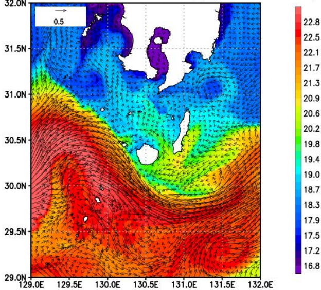
図1. 鹿児島大学工学部によって運用されている高分解能海洋モデル(DR_E)における流れ(矢印)および海面水温(赤~紫)の4月3日の結果(ホームページより引用).
